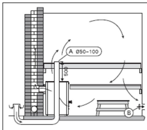
4. ábra. Mechanikai szellőztetés
