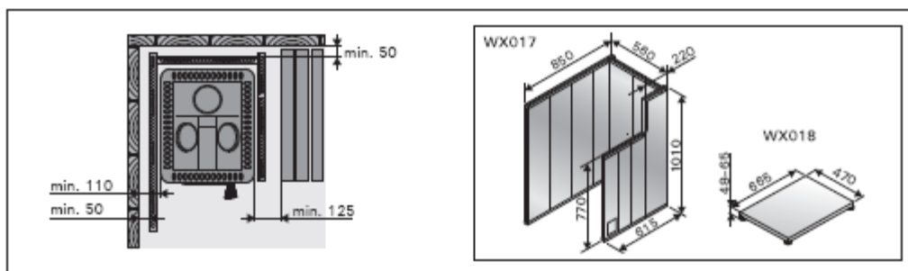
8. ábra. Harvia védőburkolat és védőalátét. (minden méret milliméterben van megadva)
