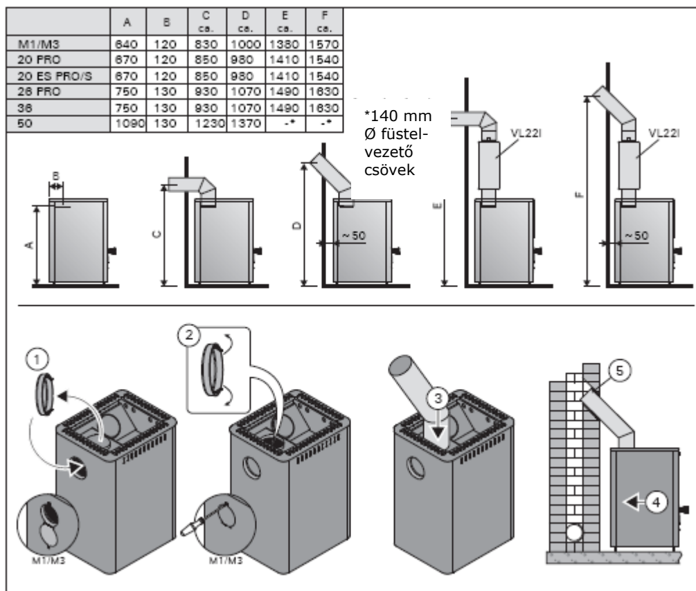
10. ábra. A kályha téglakéményhez történő csatlakoztatása a felső csatlakozó nyíláson keresztül
