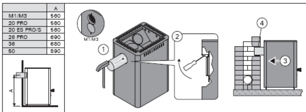
9. ábra. A kályha téglakéményhez történő csatlakoztatása a hátsó csatlakozó nyíláson keresztül
