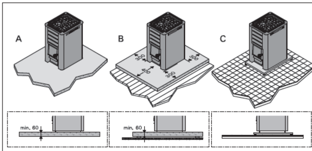
5. ábra. A padlózat védelme. (minden méret milliméterben van megadva)
