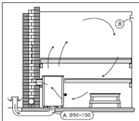
3. ábra. Gravitációs szellőzés
