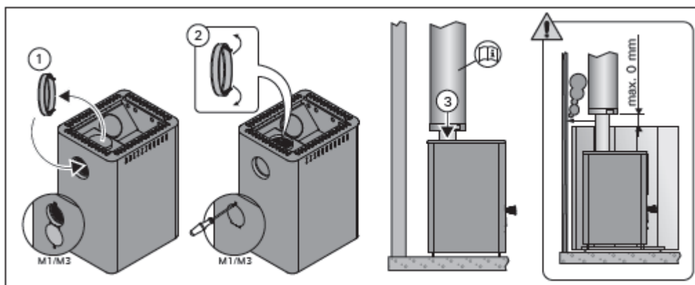
11. ábra. A kályha Harvia acélkéményhez történő csatlakoztatása. (minden méret milliméterben van megadva)
