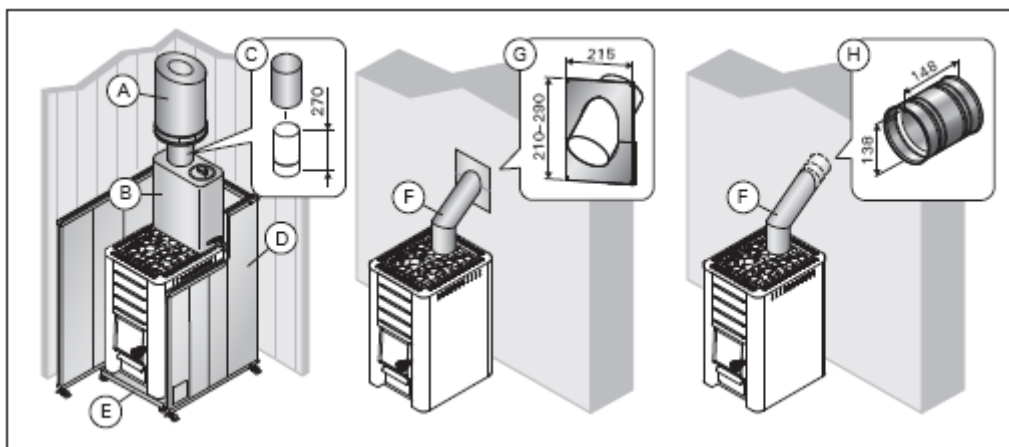
13. ábra. Kiegészítők. (minden méret milliméterben van megadva)
