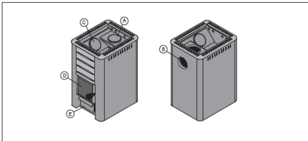
1. ábra. A kályha részei
