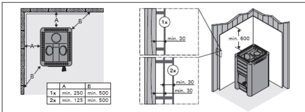
7. ábra. Védőburkolatok. (minden méret milliméterben van megadva)
