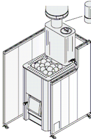
HARVIA M1/M3 FÜSTCSŐRE SZERELT VÍZMELEGÍTŐVEL ÉS HŐVÉDŐ LEMEZSEL
