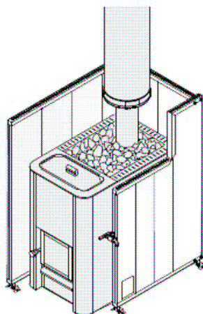
HARVIA 20 ES PRO HŐVÉDŐ LEMEZSEL
