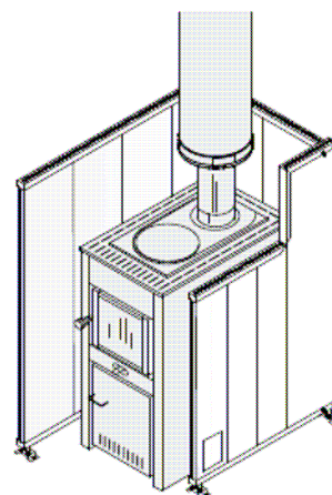
HARVIA 10 VASKÁLYHA HŐVÉDŐ LEMEZSEL
